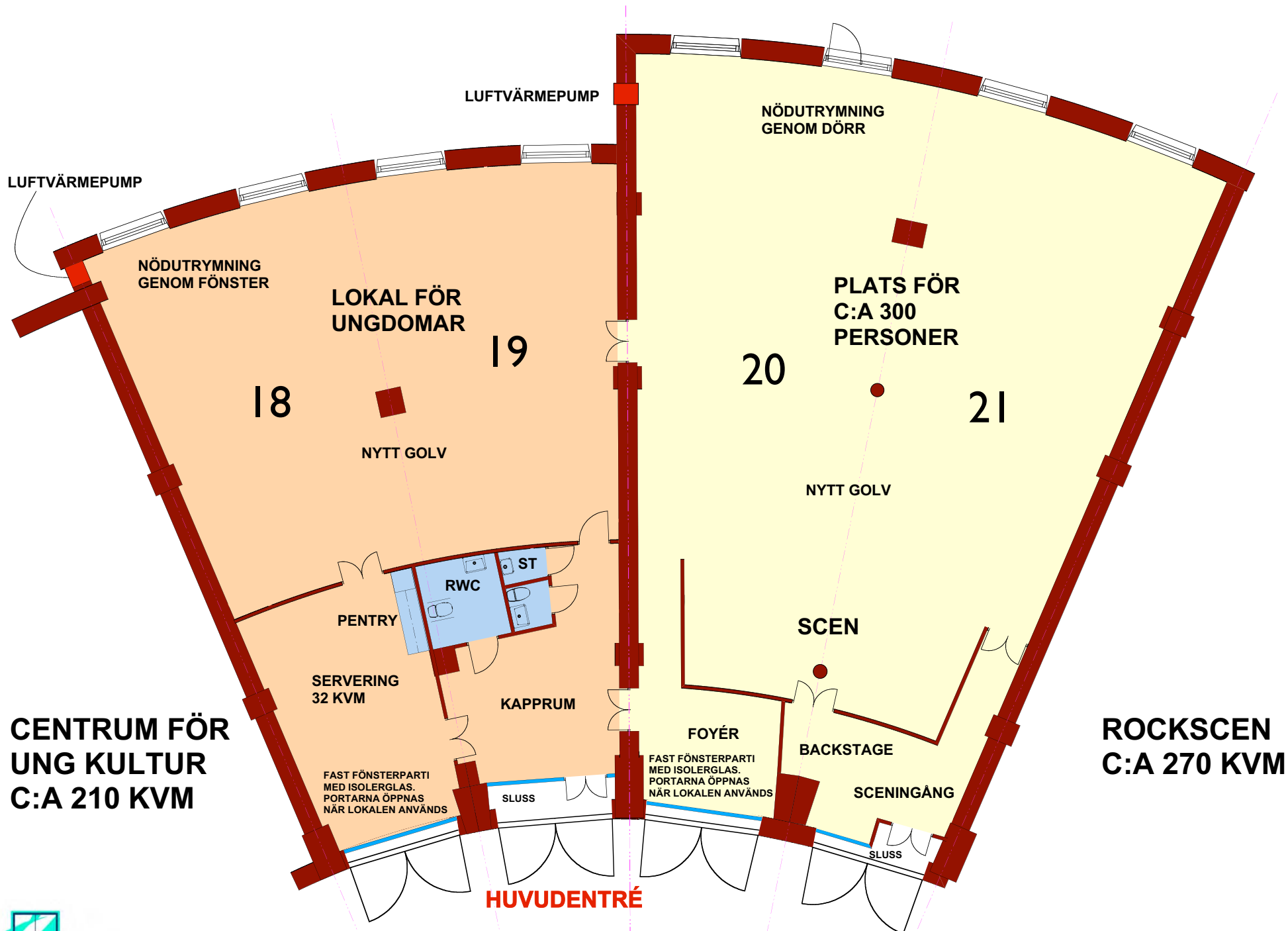
LOKSTALLARNA – KATRINEHOLMS NYA ARENA FÖR UNGDOMSKULTUR SKISS 2009.12.01
